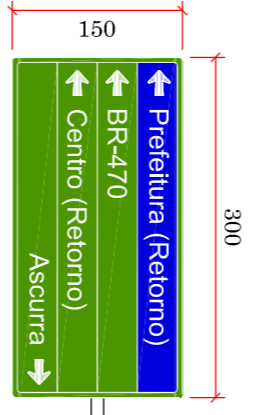
DETALHE DE PLACA SUSPensa EM SEMI-PORTICO - ALTA
