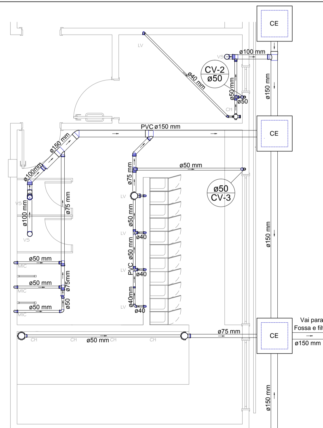
DETALHE S 02 1:50
