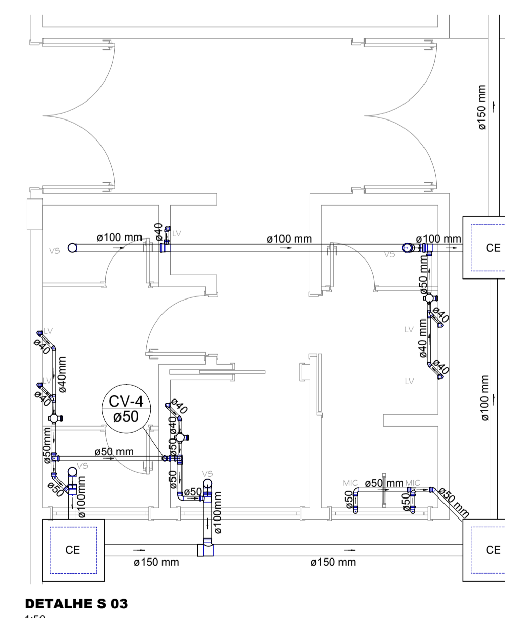
DETALHE S 03 1:50
