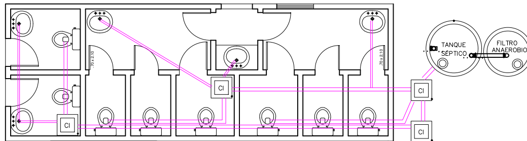
PLANTA DO SISTEMA DE ESGOTO (SANITÁRIO)
