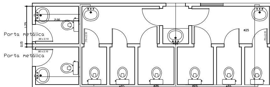
DIAGRAMA EM PLANTA (Hidraulico) ESC.: 1 : 50
