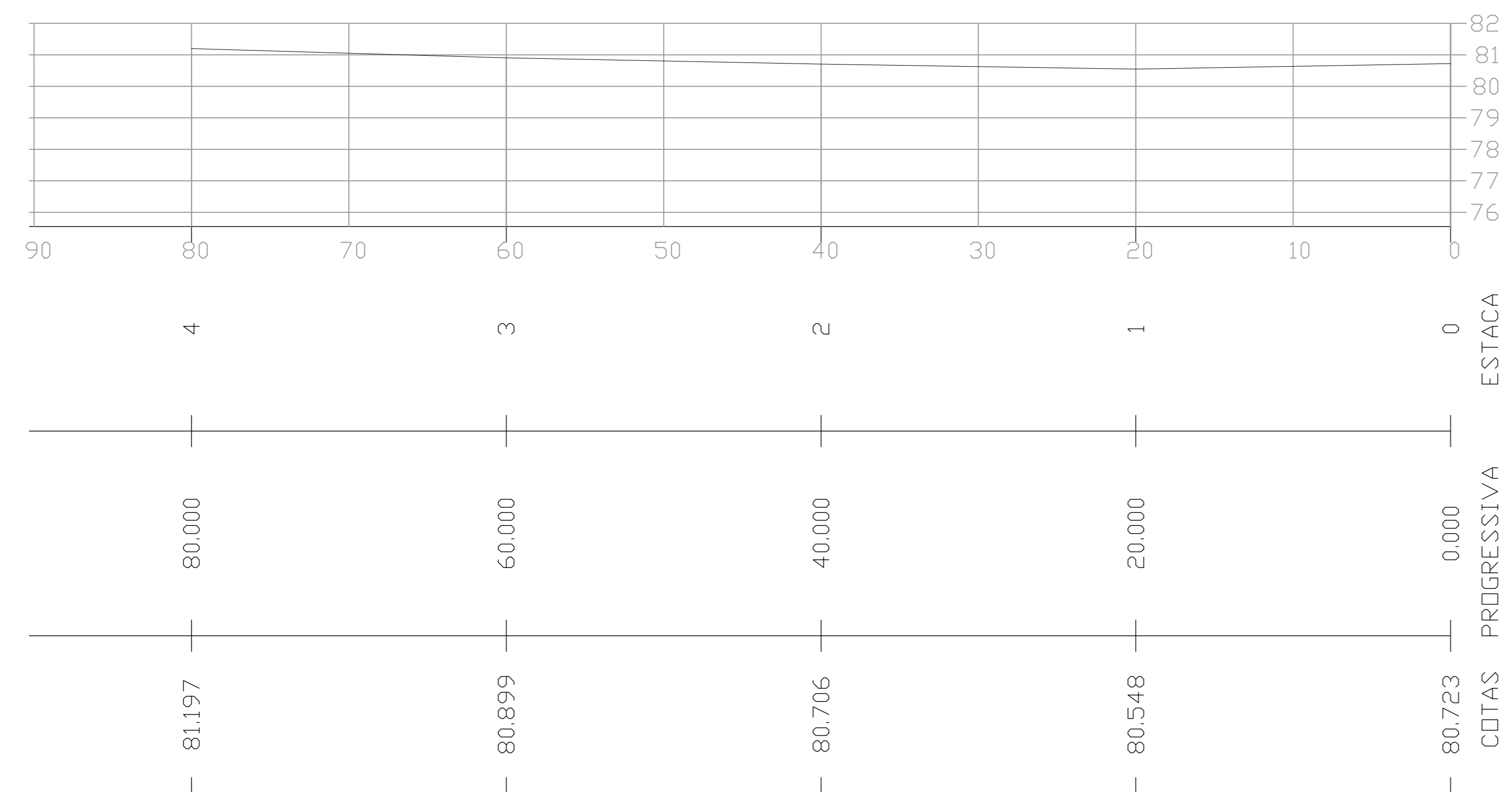
PERFIL LONGITUDINAL – EIXO DA RUA
