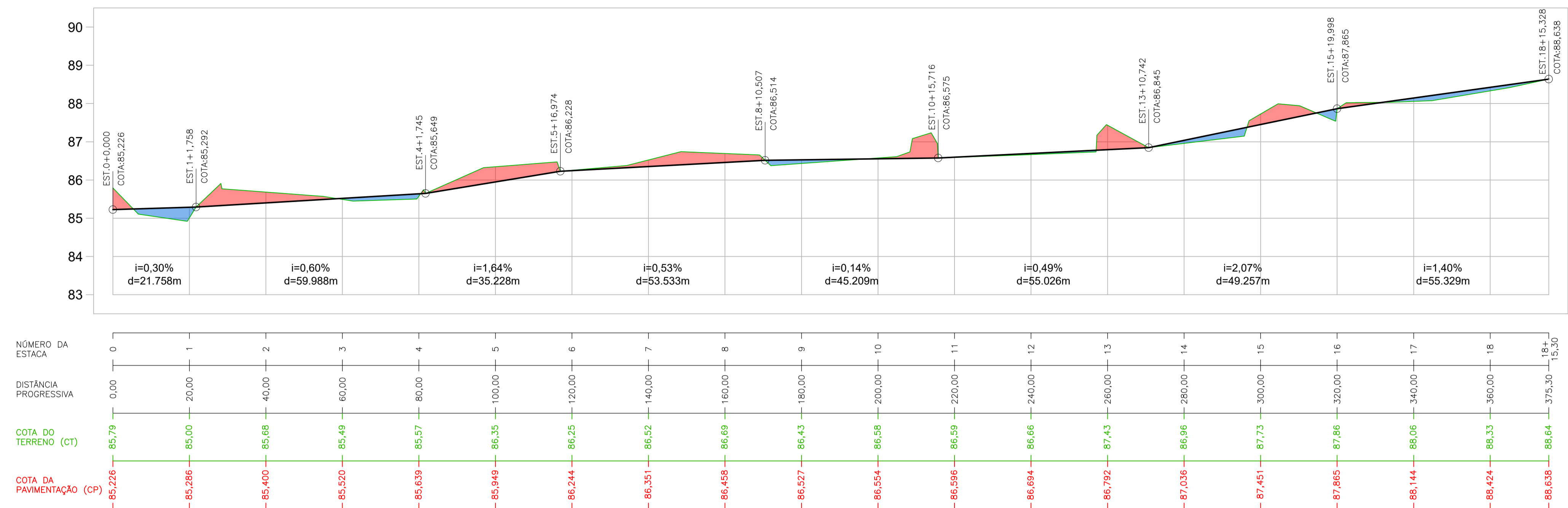
PERFIL LONGITUDINAL - EIXO DA RUA ESC.: 1/750
