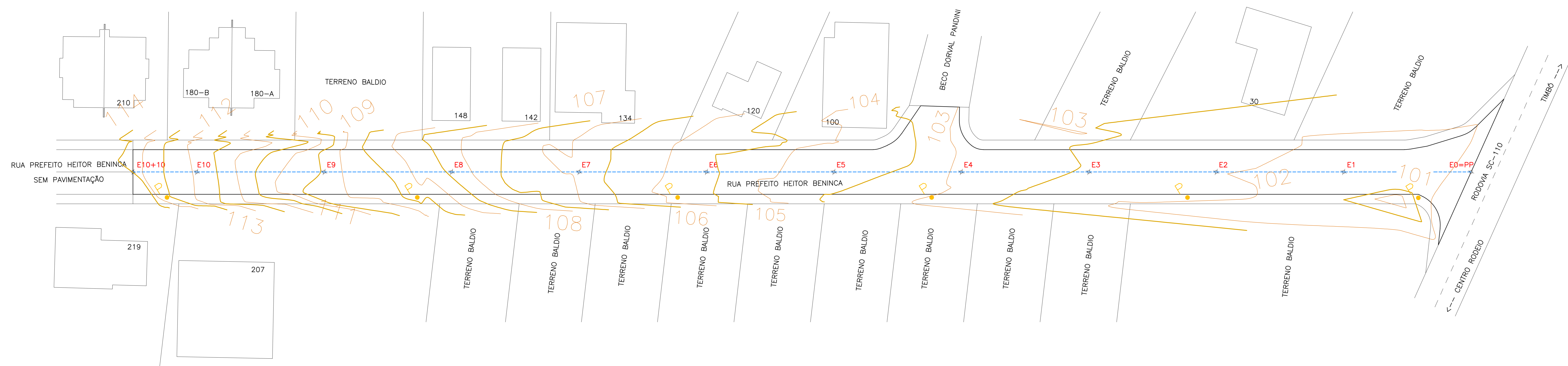
LEVANTAMENTO PLANIALTIMÉTRICO
