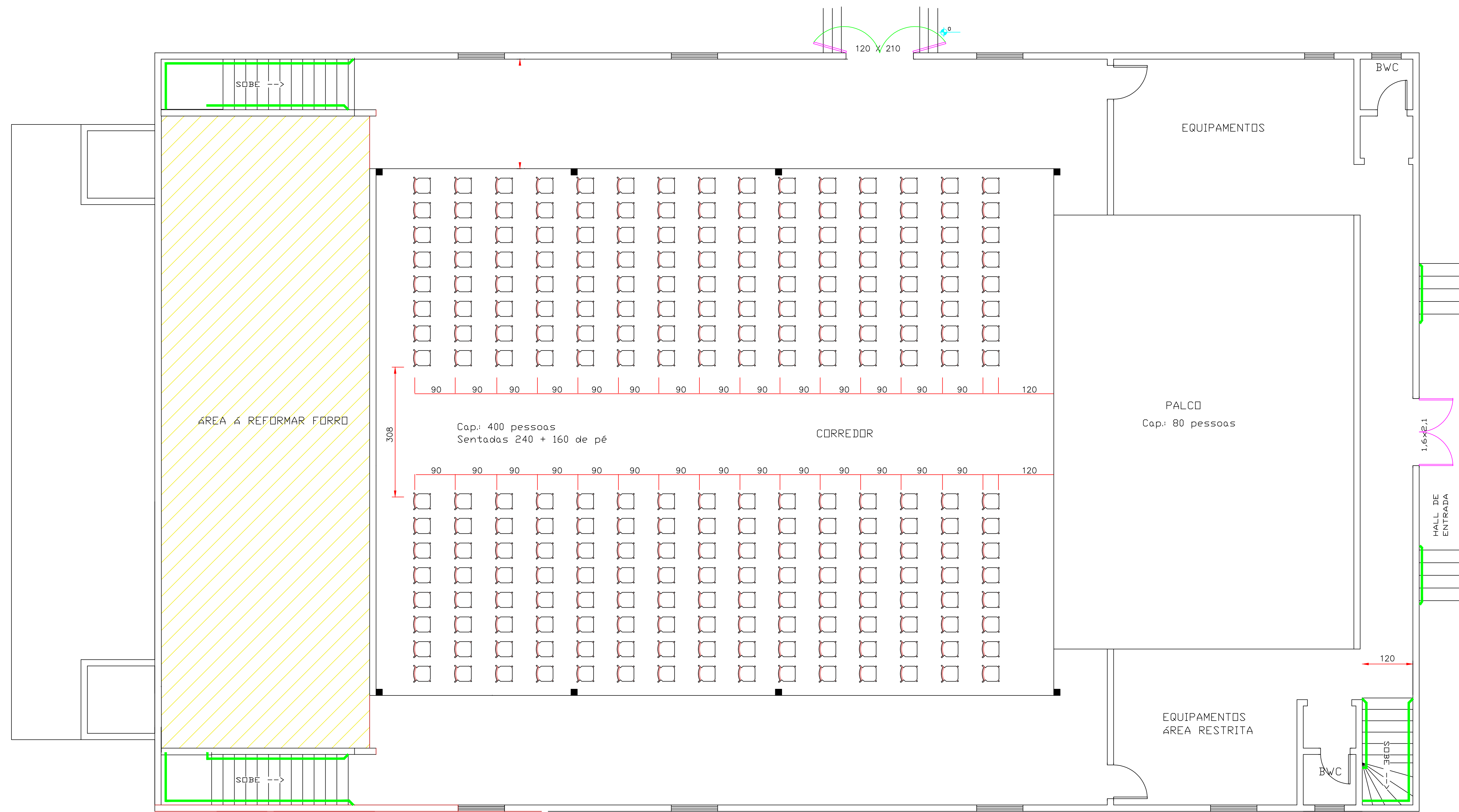
Locação da Obra ESC.1/50
